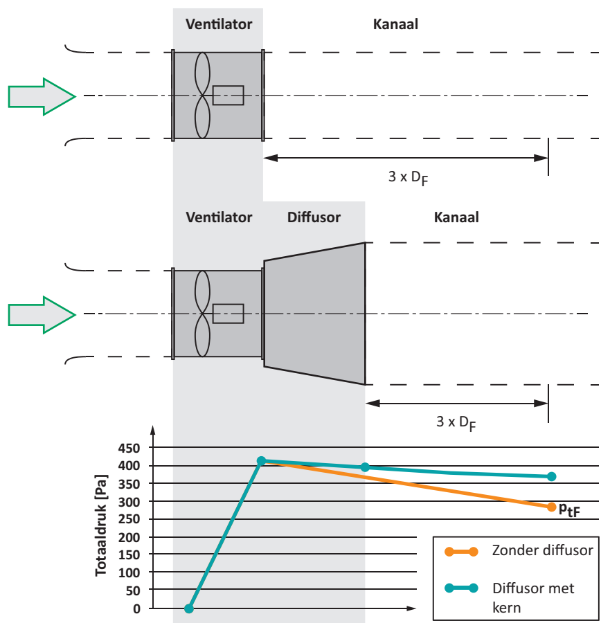
Voorbeeld drukverlies
