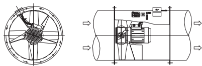
Fig. 7. Kanaal montage
