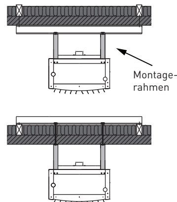
Abb. 5. Deckenmontage
