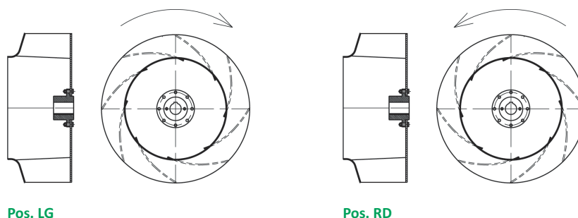
Ventilatorhjulpositioner
