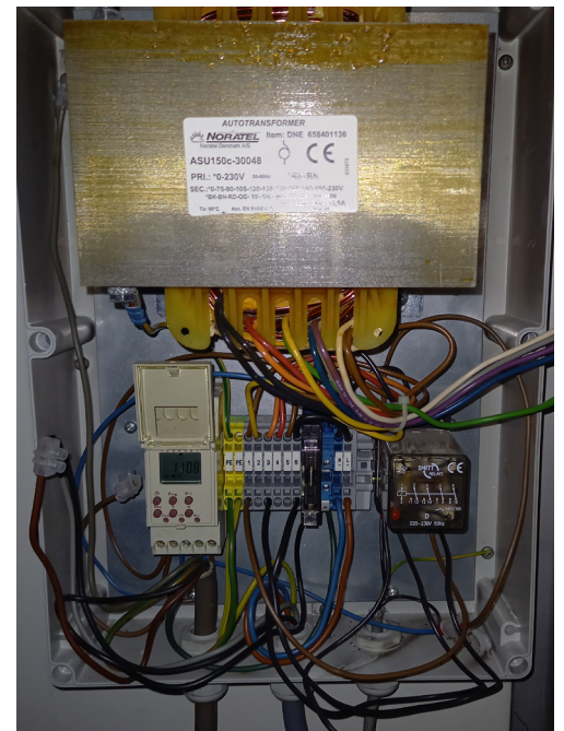
Transformator regeling oude systeem
