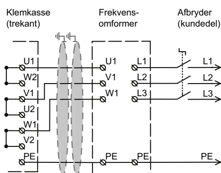
Figur 16. Klemkasse trekant-tilslutning
