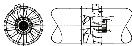
Figur 8. Montering i kanal
