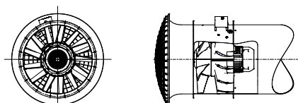
Figur 9. Kanalmontering med indløbstragt
