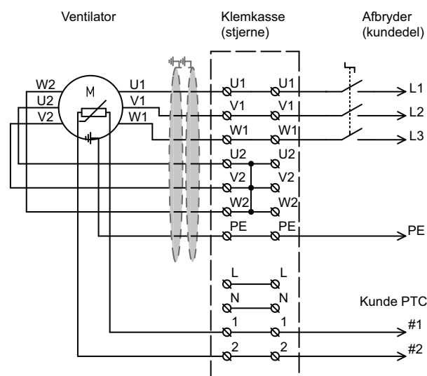
Figur 15. Klemkasse stjerne-tilslutning
