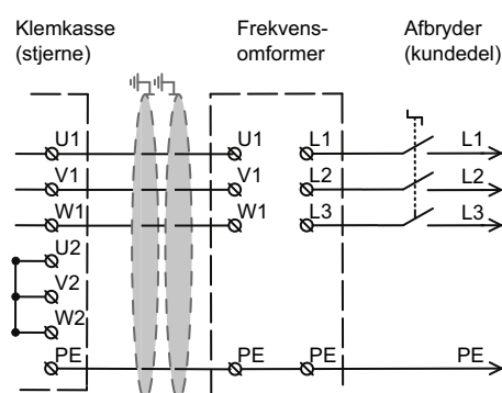
Figur 17. Klemkasse stjerne-tilslutning
