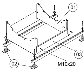
Type 3 - Horizontal fodkonsol til AZN og AZW
