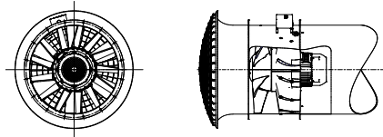
Abb. 9. Installation in Kanal mit Einlaufkonus und Schutzgitter
