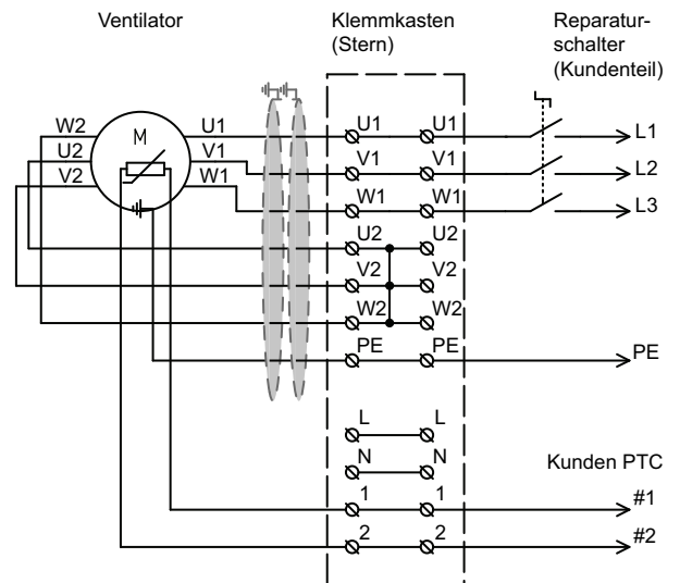
Abb. 15. Klemmenkasten-Sternschaltung
