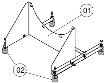
Typ 1 - Horizontaler Rahmen für AZL
