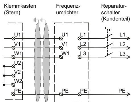
Abb. 17. Klemmenkasten-Sternschaltung
