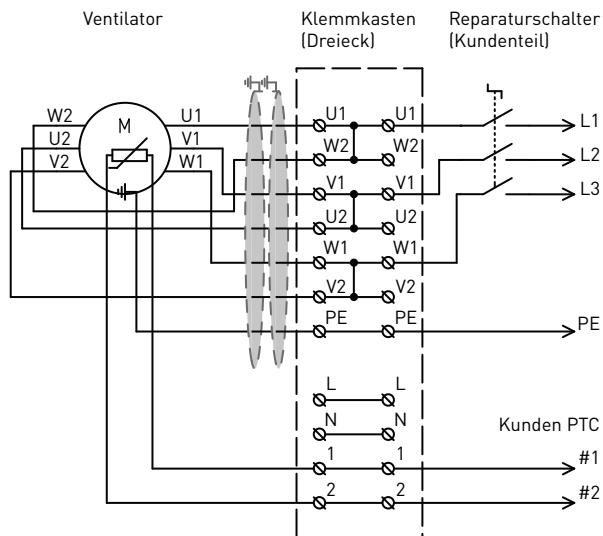
Abb. 14. Klemmenkasten-Dreieckschaltung
