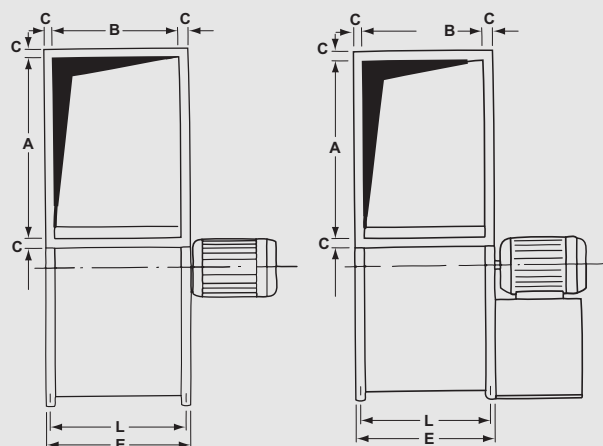
Direkte drevet CNA 250, -315, -400 CNB 400
