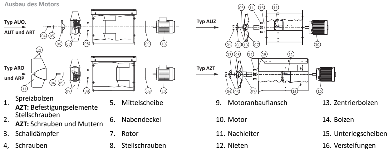
Abbildung 8. Hauptkomponenten
